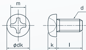
(+)なべ小ねじ
